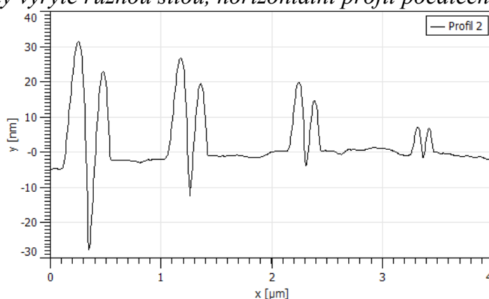
Obr. 10: Rýhy vyryté různou silou, horizontální profil střední části rýh
