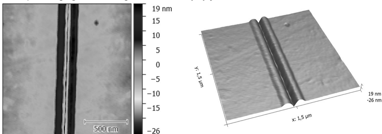
Obr. 13: Referenční rýha, 2D a 3D topografická mapa (vpravo)
