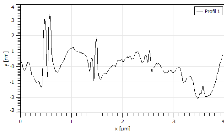
Obr. 12: Rýhy vyryté různou silou, horizontální profil střední části rýh
