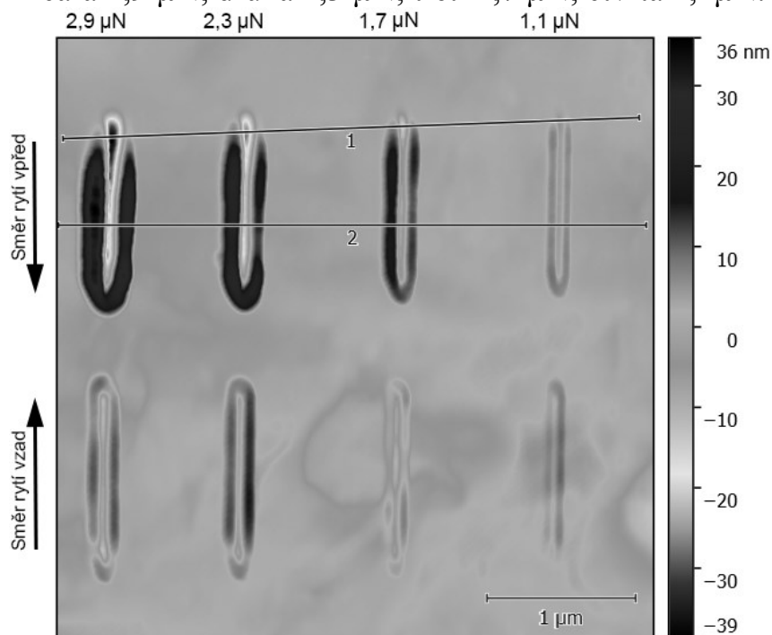
Obr. 8: Rýhy vyryté různou silou, topografická mapa ( 4 \times 4 \mu\text{m} )
