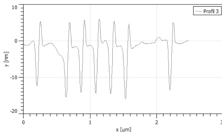
Obr. 28: Kód - slovo PASSWORD ve dvojkové soustavě, horizontální profil prvního řádku (v místě největší hloubky)
