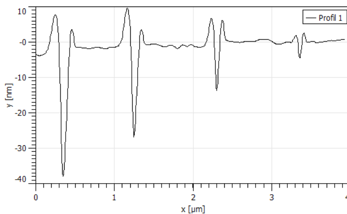
Obr. 9: Rýhy vyryté různou silou, horizontální profil počáteční části rýh
