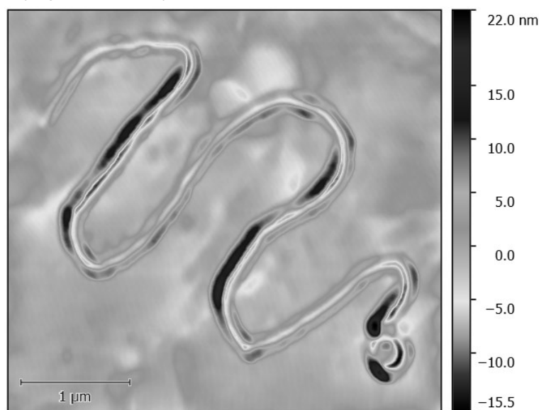
Obr. 7: Had, topografická mapa (4 x 4 μm)
