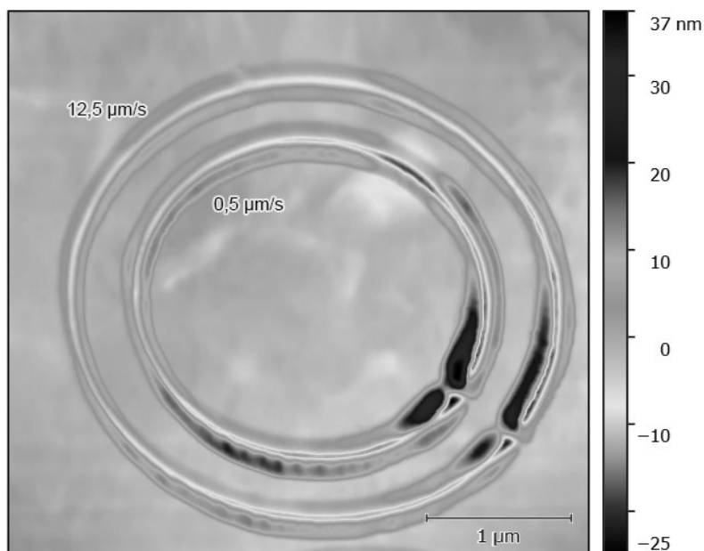
Obr. 3: Kruhy vytvořené různými rychlostmi, topografická mapa (4 x 4 μm)
