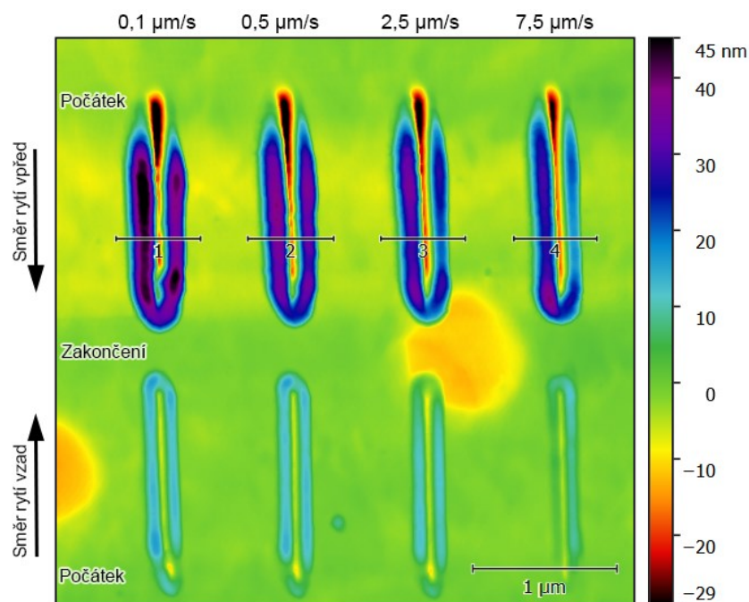
Obr. 1: Rýhy vytvořené různými rychlostmi, topografická mapa (4 x 4 μm)
