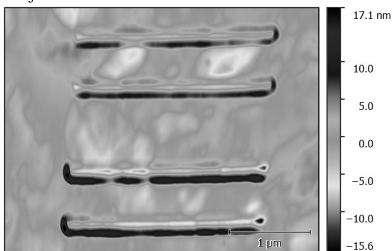
Obr. 6: Rýhy vyryté do stran, topografická mapa (4 x 3 μm)
