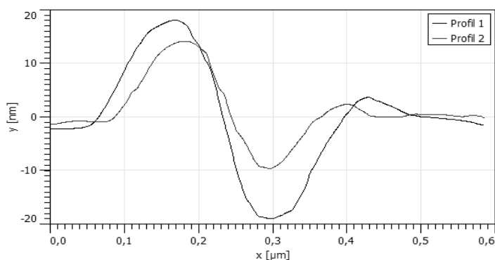
Obr. 32: Kód – slovo PASSWORD v trojkové soustavě, porovnání vertikálního profilu menší a větší rýhy
