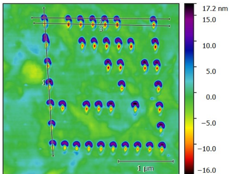
Obr. 23: Kód – slovo PASSWORD ve dvojkové soustavě, topografická mapa (3,2 x 3,2 \mu\text{m} )
