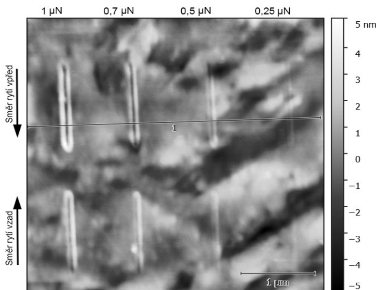
Obr. 11: Rýhy vyryté různou silou, topografická mapa (4 x 4 \mu\text{m} )
