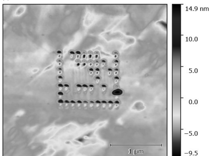
Obr. 29: Kód – slovo PASSWORD ve dvojkové soustavě (zmenšená verze), topografická mapa (3,2 x 3,2 μm)
