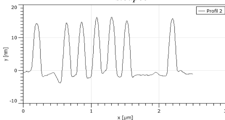
Obr. 27: Kód - slovo PASSWORD ve dvojkové soustavě, horizontální profil prvního řádku
