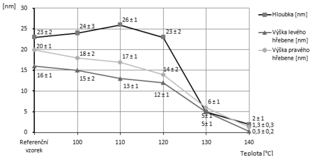
Obr. 15: Porovnání rozměrů rýh vystavených různým teplotám po dobu 15 minut.
