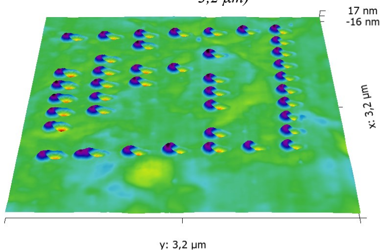
Obr. 25: Kód - slovo PASSWORD ve dvojkové soustavě, 3D topografická mapa (3,2 x 3,2 \mu\text{m} ), pohled ze strany
