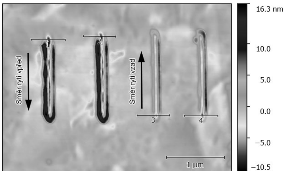
Obr. 5: Rýhy vyryté směrem vpřed a vzad, topografická mapa (4 x 3 μm)
