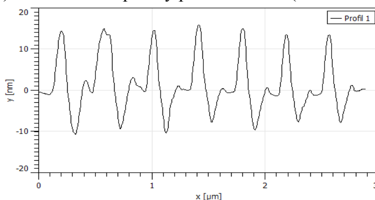
Obr. 26: Kód - slovo PASSWORD ve dvojkové soustavě, vertikální profil prvního sloupce
