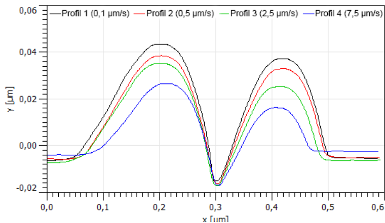
Obr. 2: Rýhy vytvořené různými rychlostmi, horizontální profily středních částí rýh
