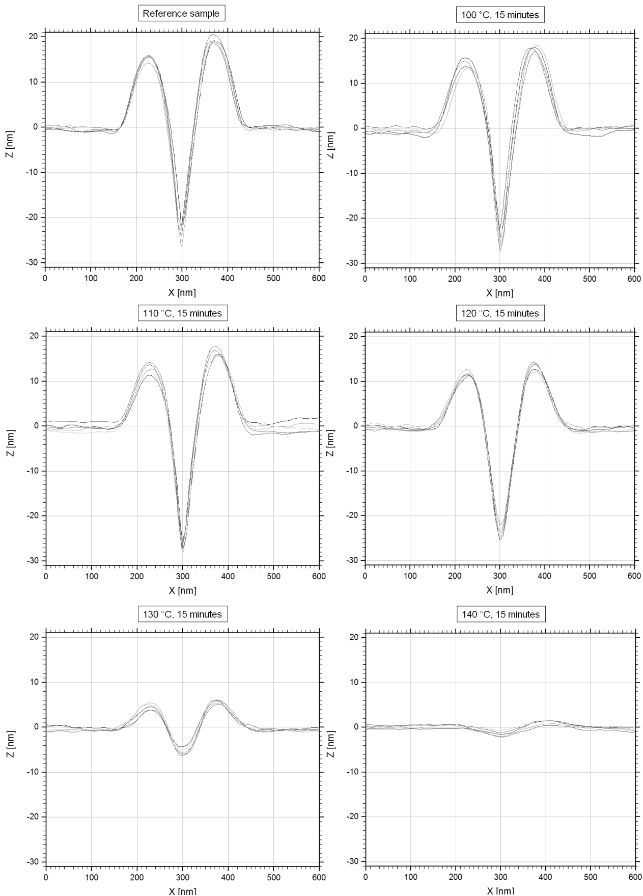
Obr. 14: Profily rýh vystavených zvýšeným teplotám po dobu 15 minut.
