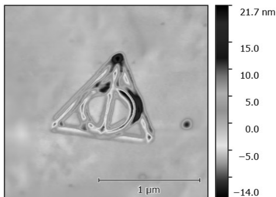
Obr. 19: Symbol – trojúhelník (zmenšený), topografická mapa ( 2 \times 2 \mu\text{m} )
