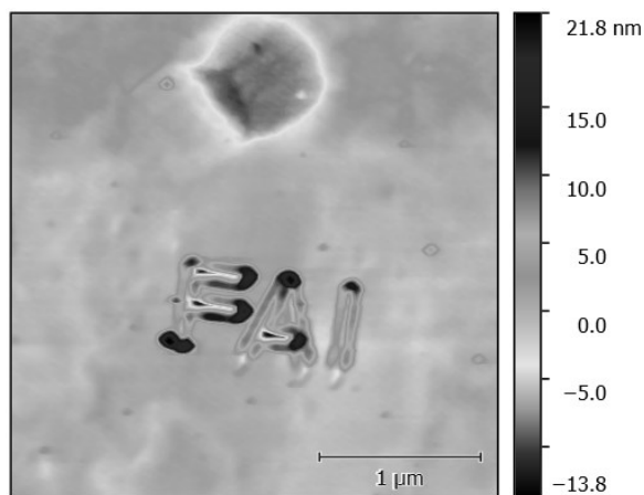
Obr. 22: Nápis FAI (zmenšený), topografická mapa ( 3 \times 3 \mu\text{m} )
